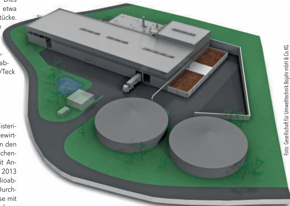
Die Grafik zeigt eine geplante Bioabfallvergärungsanlage in Zuffenhausen.
